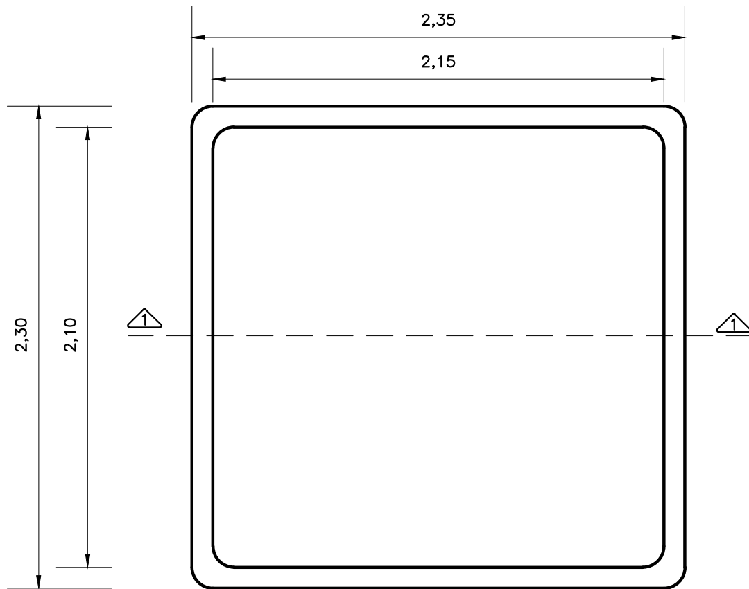
PLANTA – DIMENSÕES
