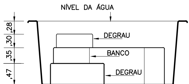
CORTE 3
