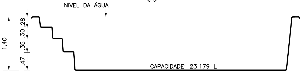
CORTE 1
