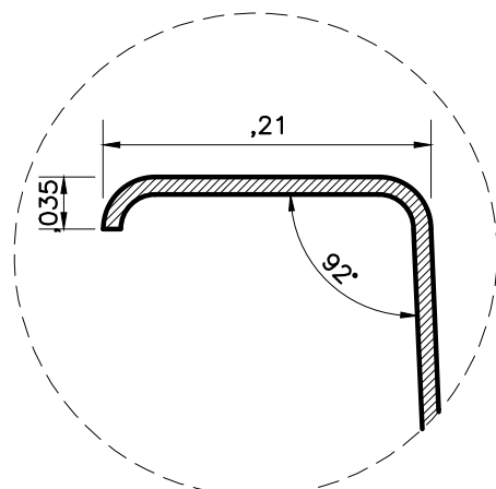
DETALHE BORDA
