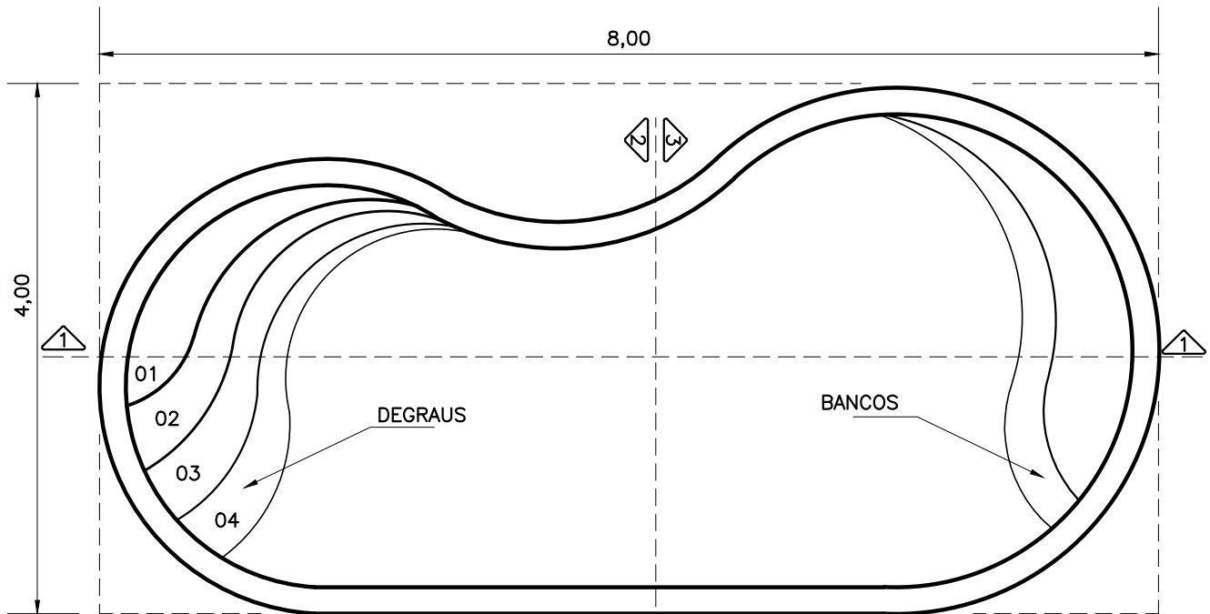
NÍVEL DA ÁGUA PLANTA - DIMENSÕES
