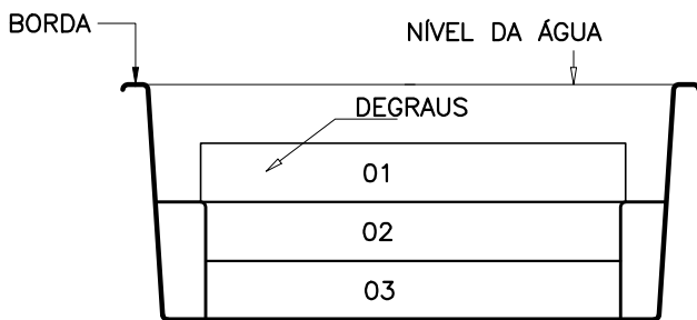
CORTE 2
