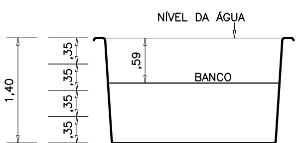
CORTE 3
