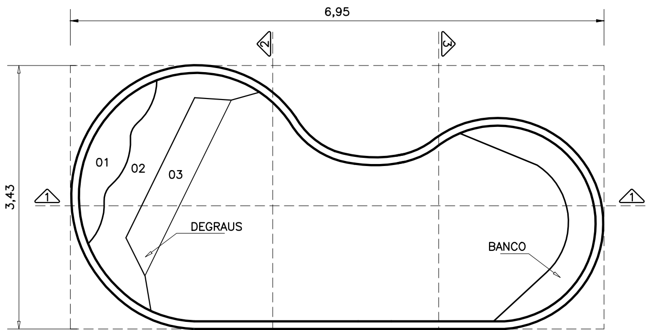
PLANTA - DIMENSÕES
