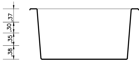
CORTE 3
