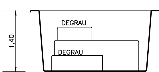
CORTE 2
