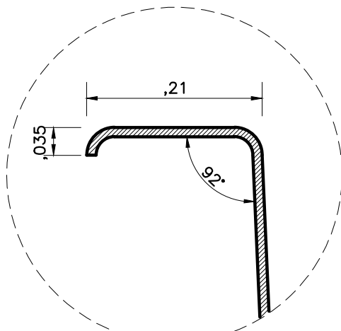
DETALHE BORDA
