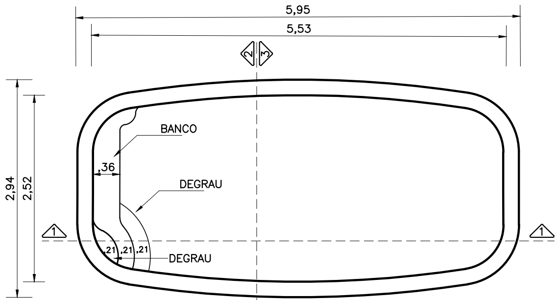
PLANTA-DIMENSÕES
