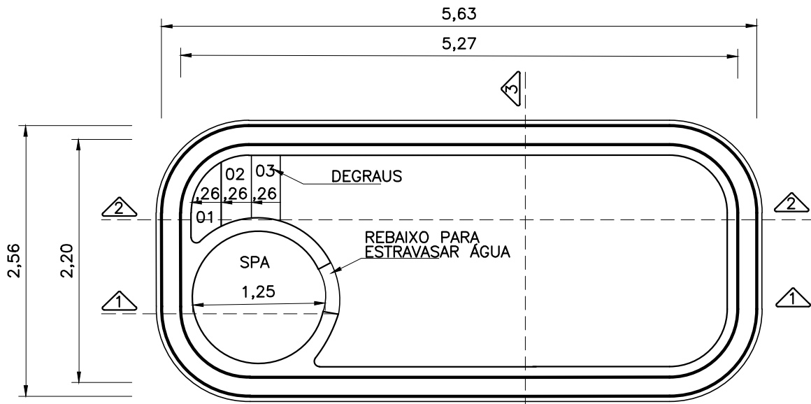
PLANTA - DIMENSÕES
