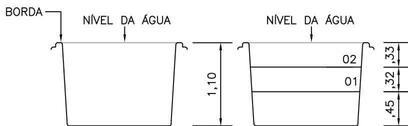
CORTE 2
