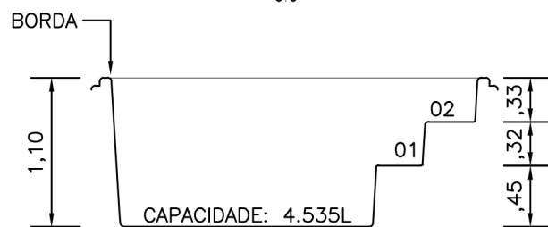
CORTE 1
