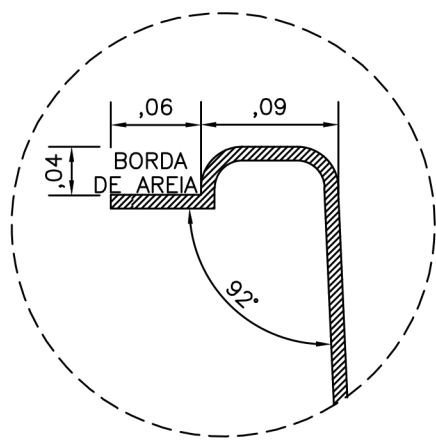
DETALHE BORDA
