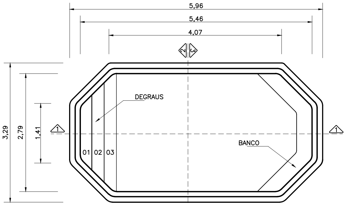
PLANTA - DIMENSÕES
