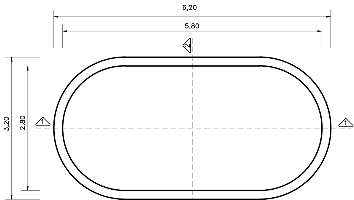
PLANTA-DIMENSÕES
