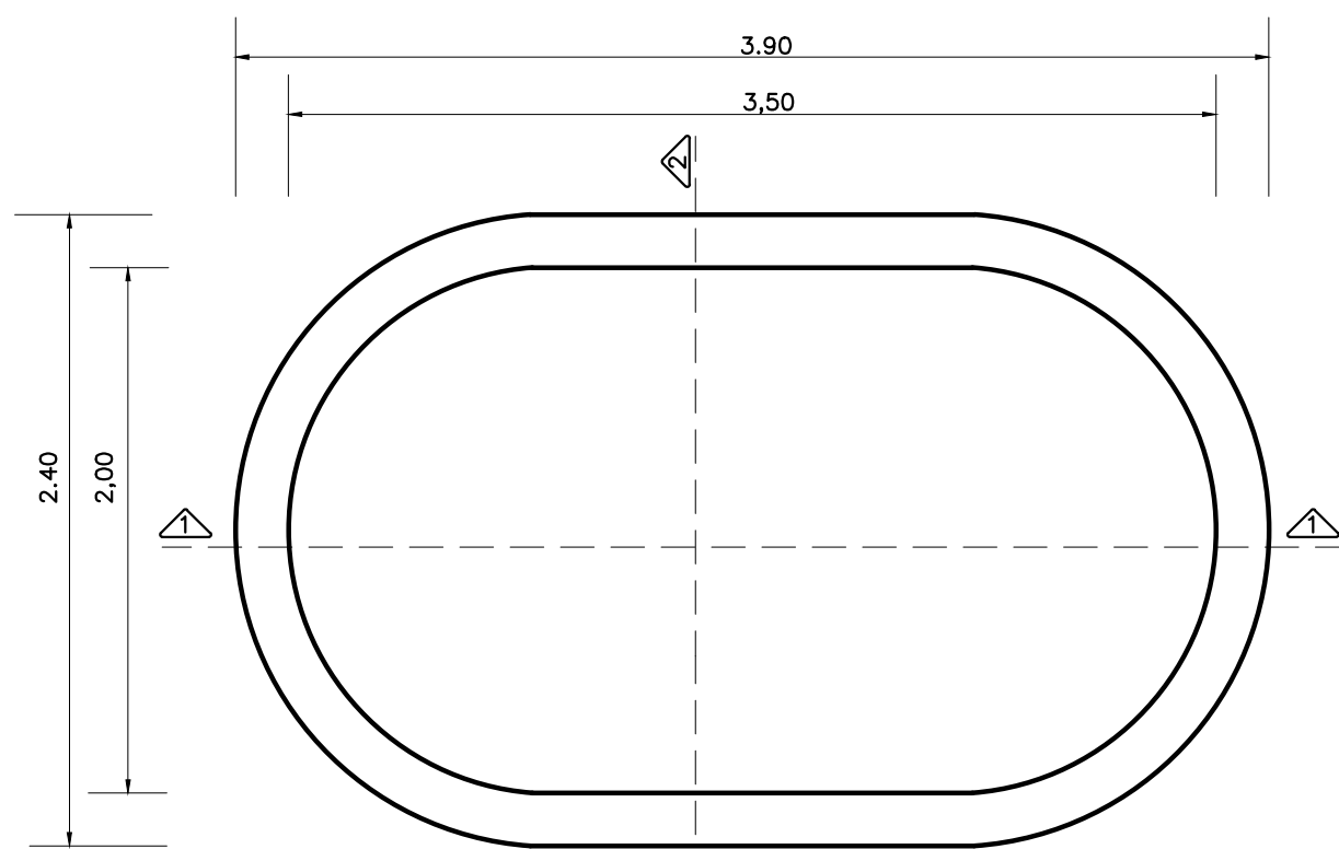
PLANTA - DIMENSÕES
