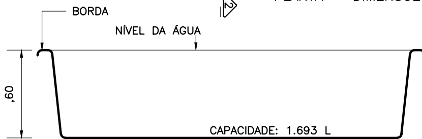
CORTE 1
