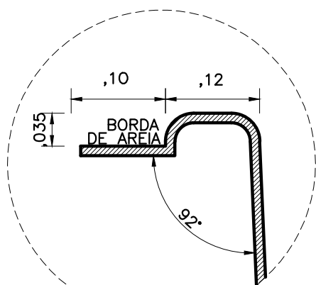
DETALHE BORDA
