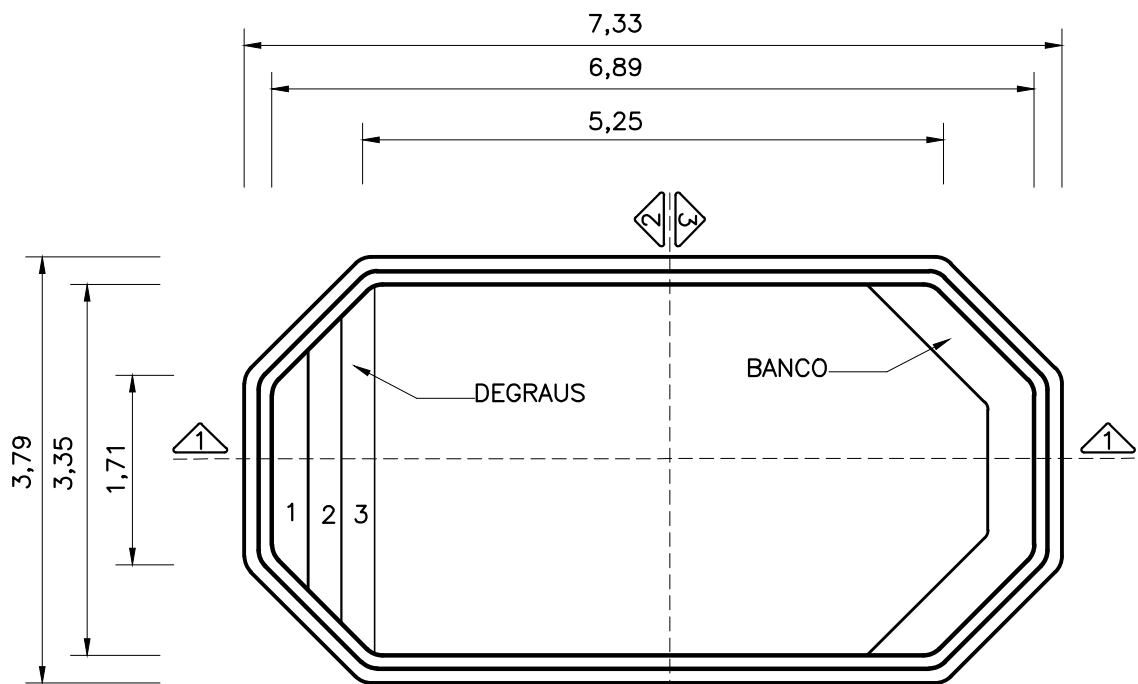
PLANTA - DIMENSÕES
