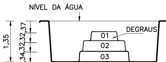
CORTE 3
