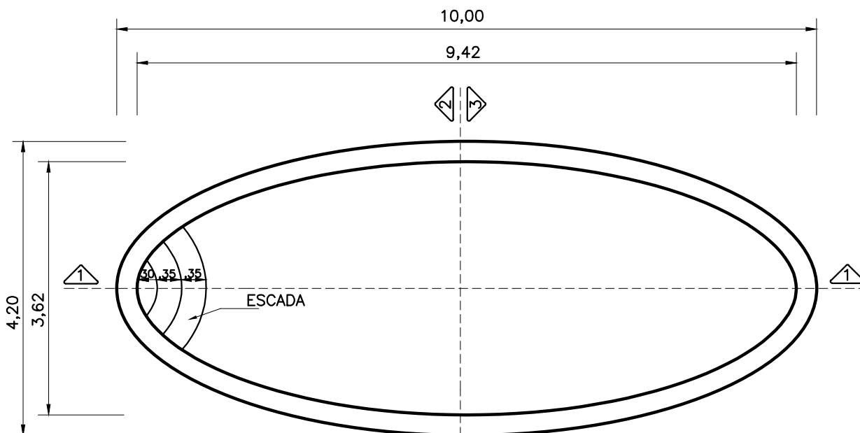
PLANTA - DIMENSÕES
