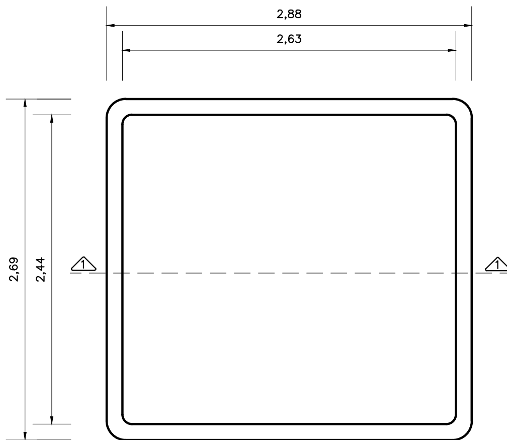
PLANTA – DIMENSÕES
