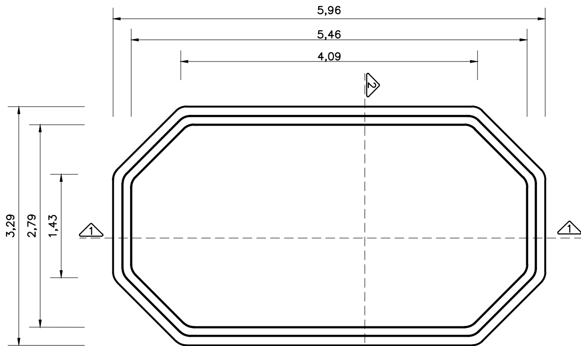
PLANTA - DIMENSÕES
