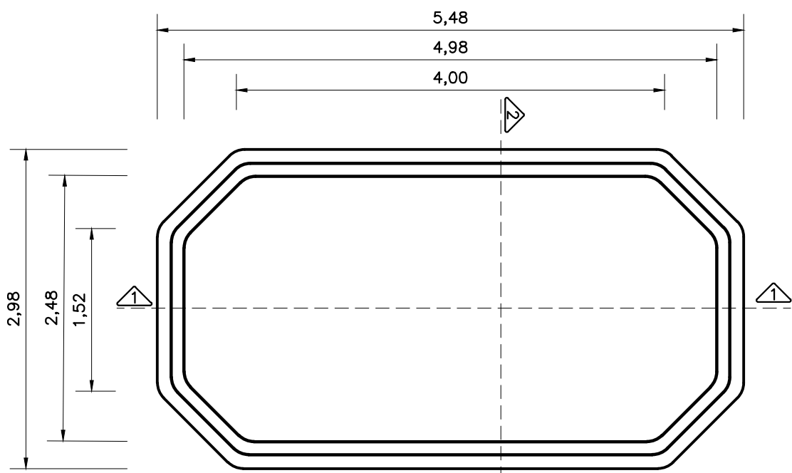
PLANTA - DIMENSÕES
