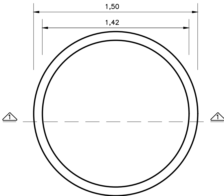
PLANTA – DIMENSÕES
