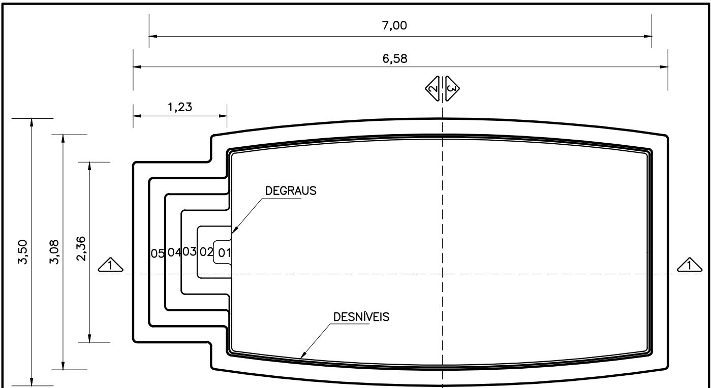
PLANTA - DIMENSÕES
