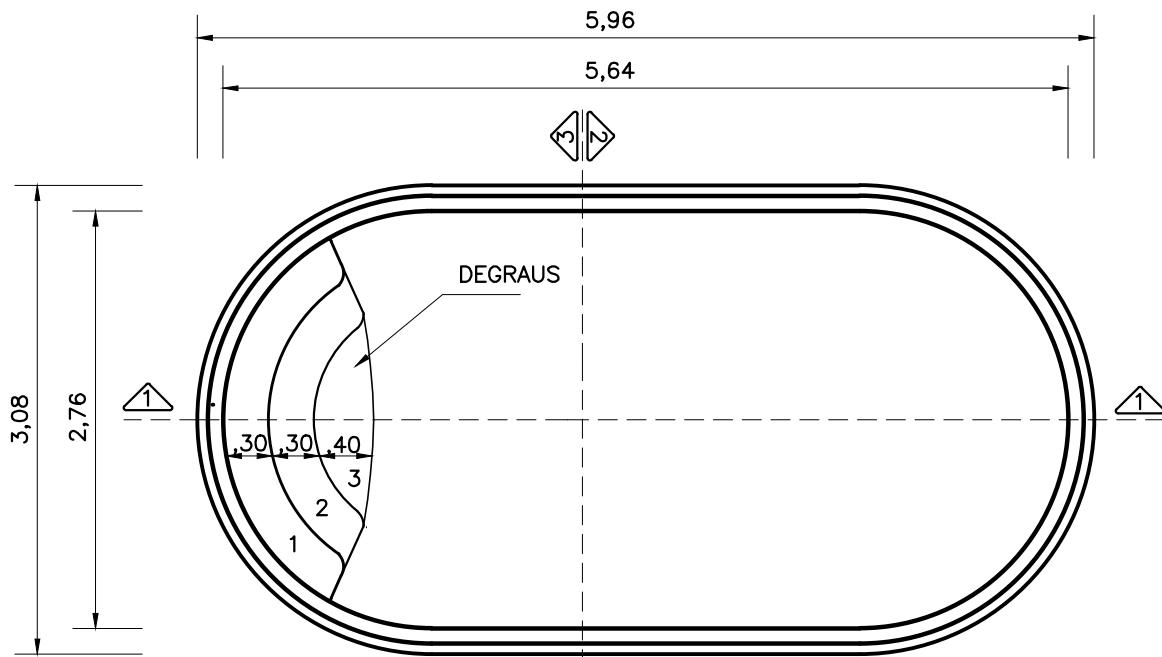
PLANTA - DIMENSÕES
