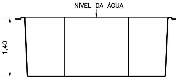
CORTE 2
