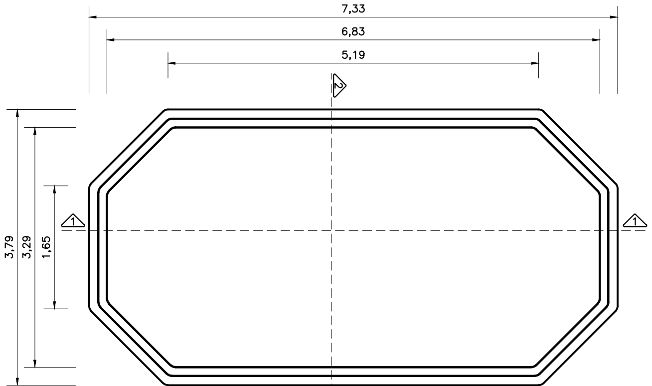
PLANTA - DIMENSÕES
