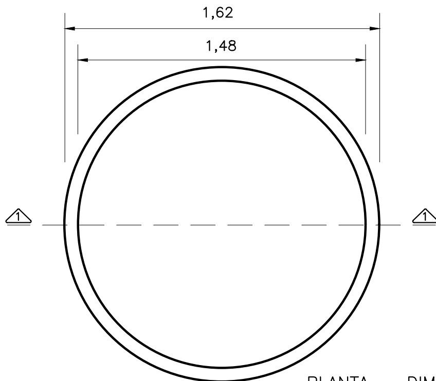
PLANTA – DIMENSÕES
