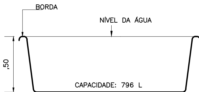
CORTE 01
