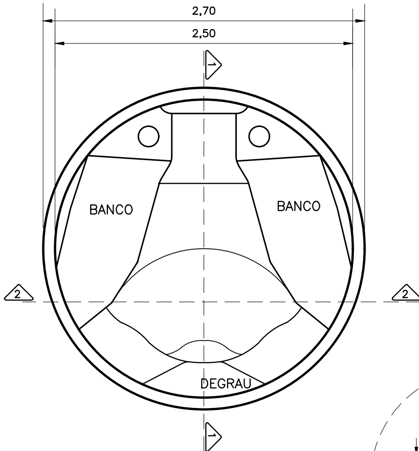
PLANTA - DIMENSÕES
