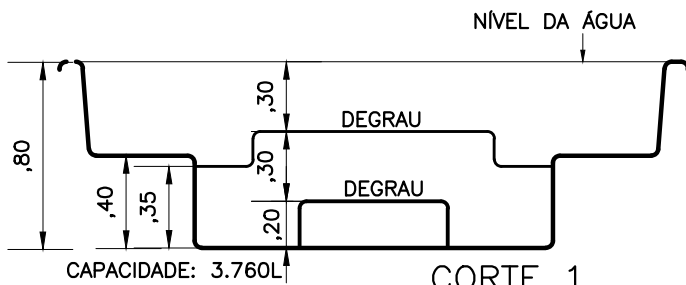
CORTE 1
