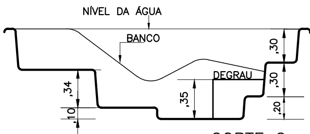
CORTE 2
