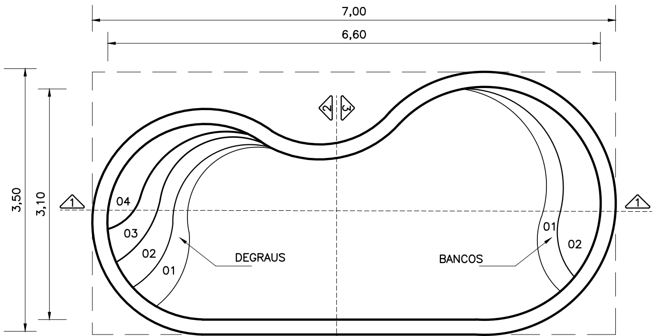
PLANTA - DIMENSÕES
