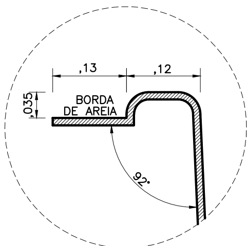
DETALHE BORDA
