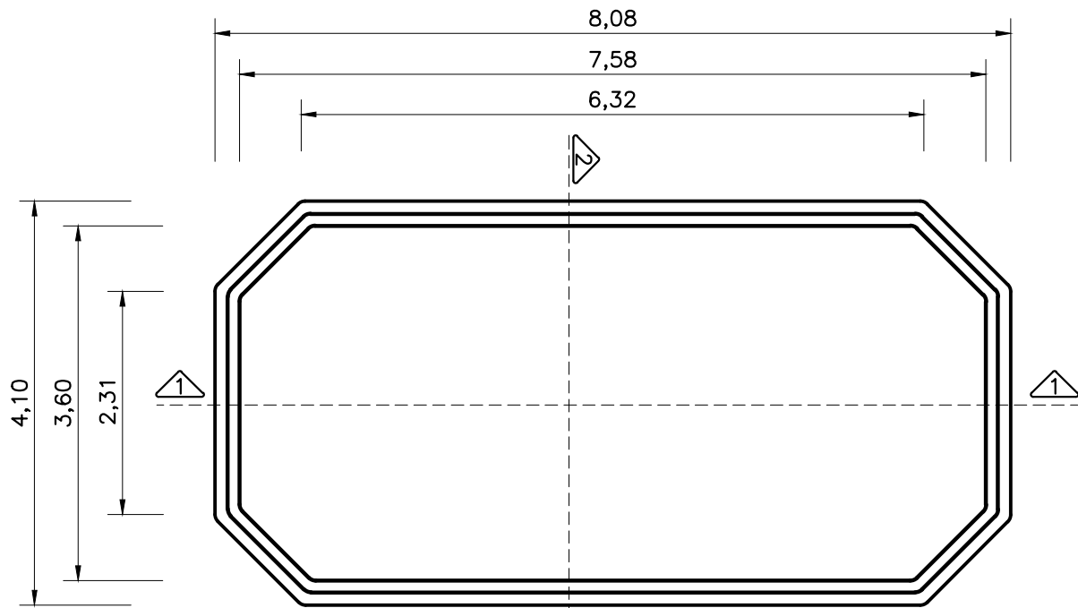
PLANTA - DIMENSÕES
