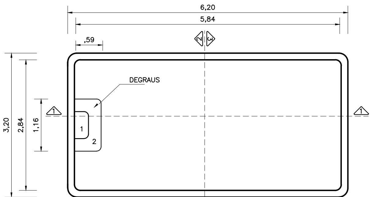
PLANTA - DIMENSÕES
