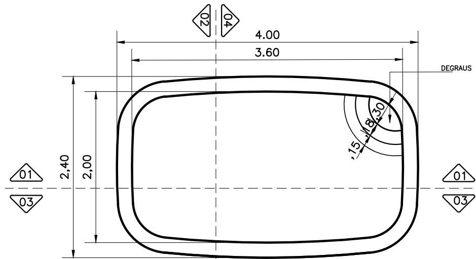
PLANTA - DIMENSÕES
