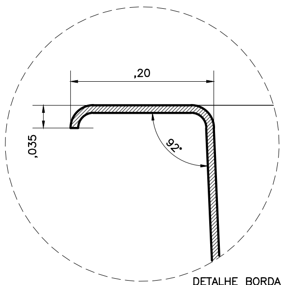
DETALHE BORDA
