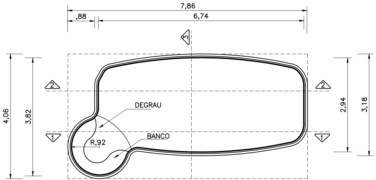
PLANTA - DIMENSÕES
