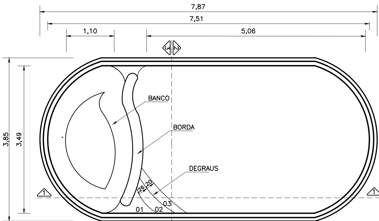
PLANTA - DIMENSÕES
