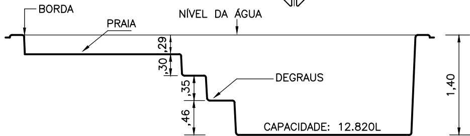
CORTE 1
