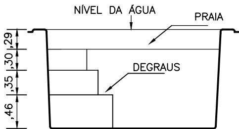
CORTE 2
